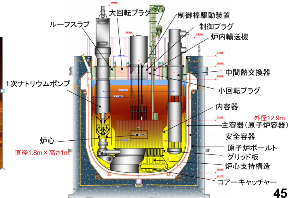
インド カルパッカムに建設中のPFBRプラント
