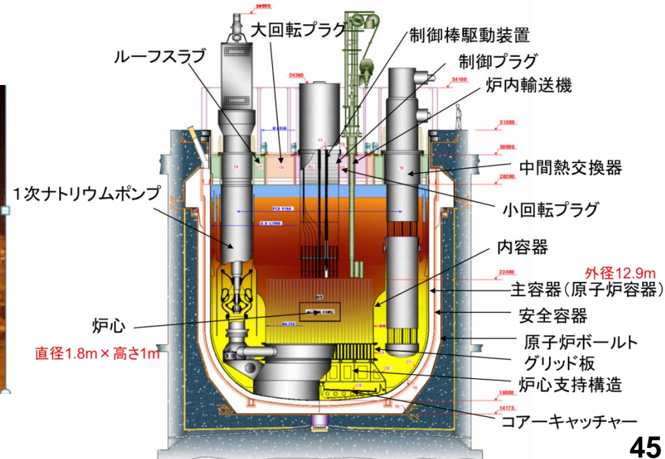
インド カルパッカムに建設中のPFBRプラント
