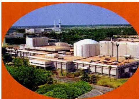
Pu-239 (FBTR)
